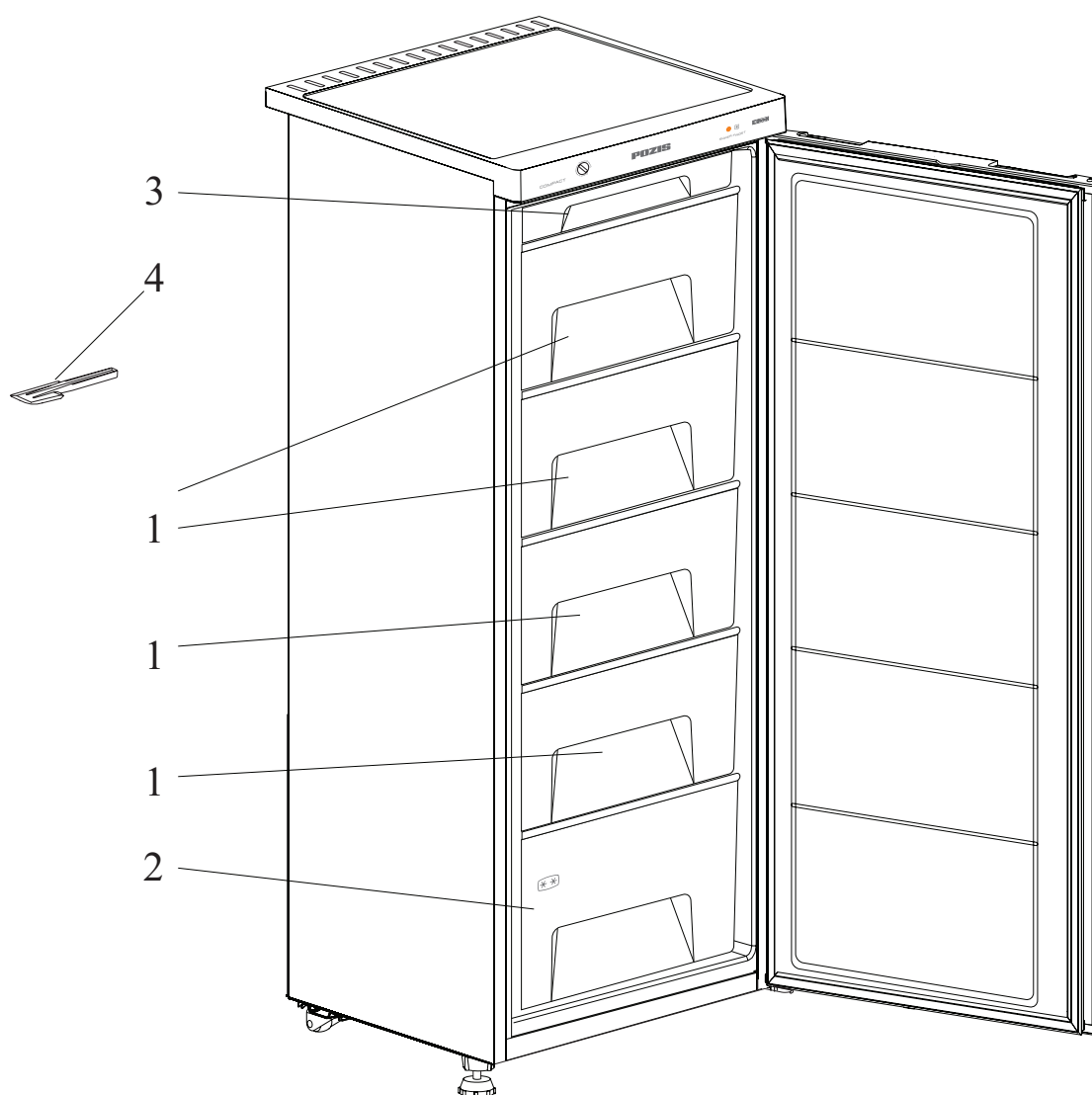
Рис. 1 Схема расположения отделений морозильника и его комплектующих Комплектация морозильника в соответствии с таблицей 2
