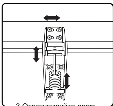
3.Отрегулируйте дверь.
